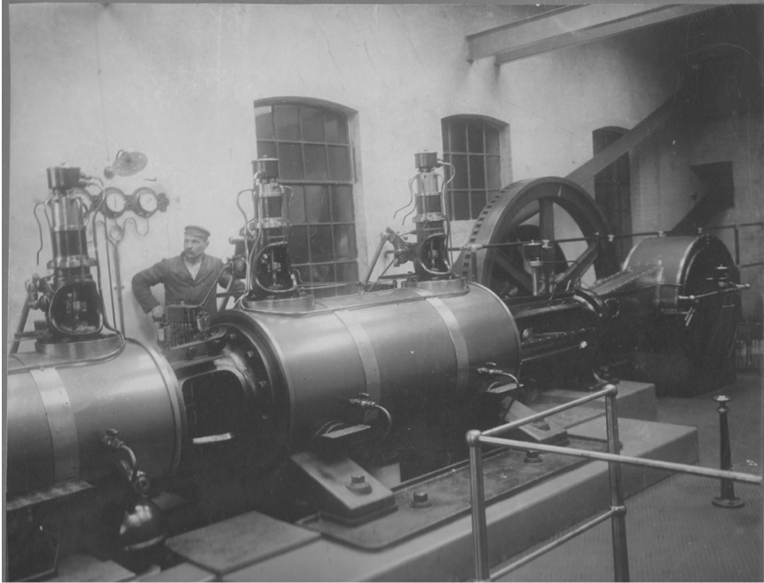
Foto: 17 Ångmaskin anskaffad 1915 [R3]
